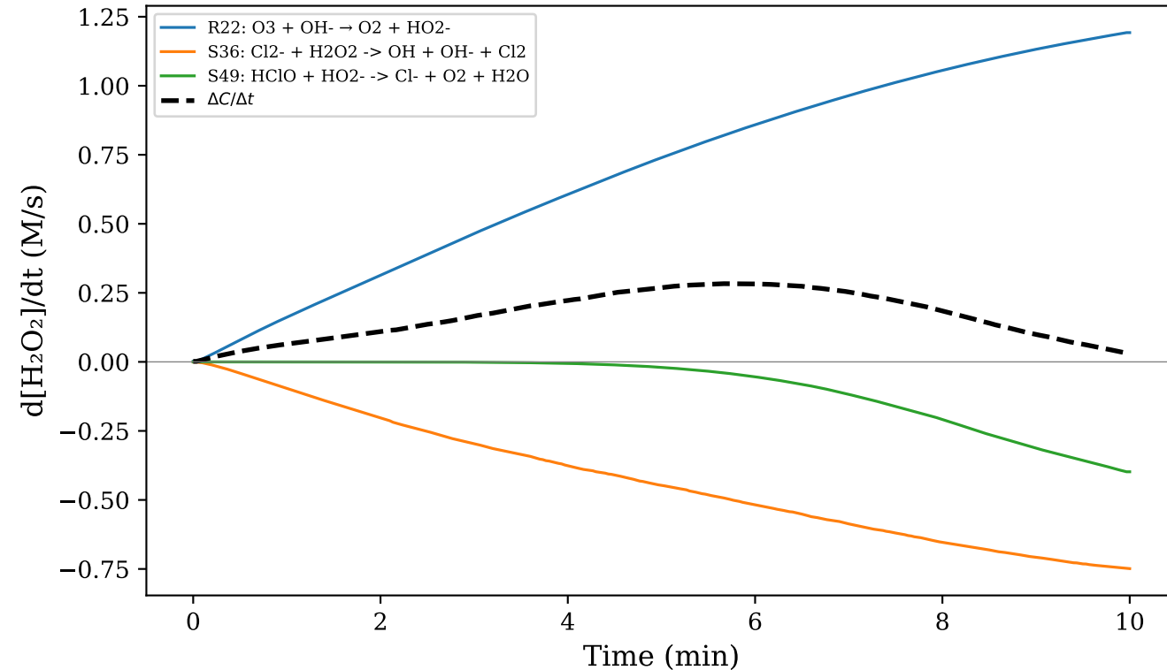
(d) \text{H}_2\text{O}_2
